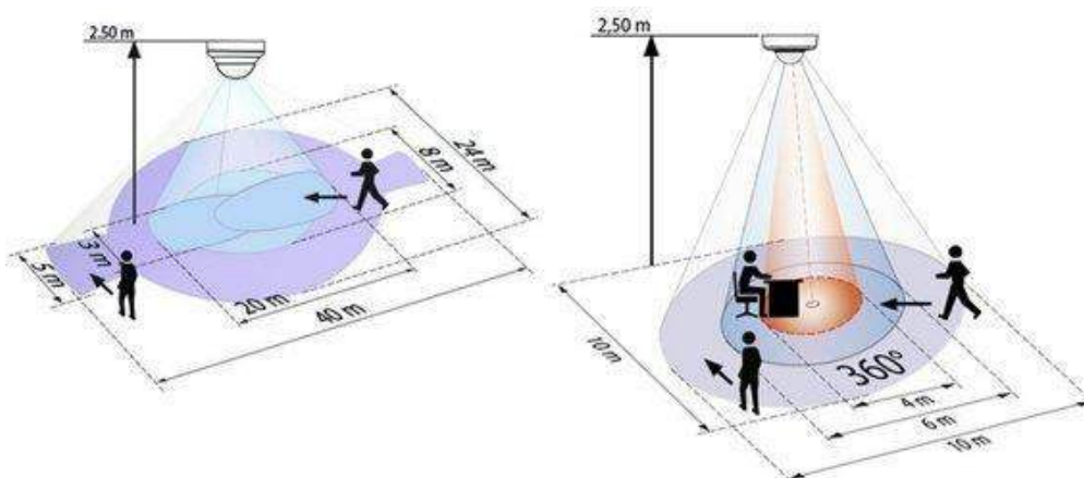
Рисунок 4 - Датчик присутствия
